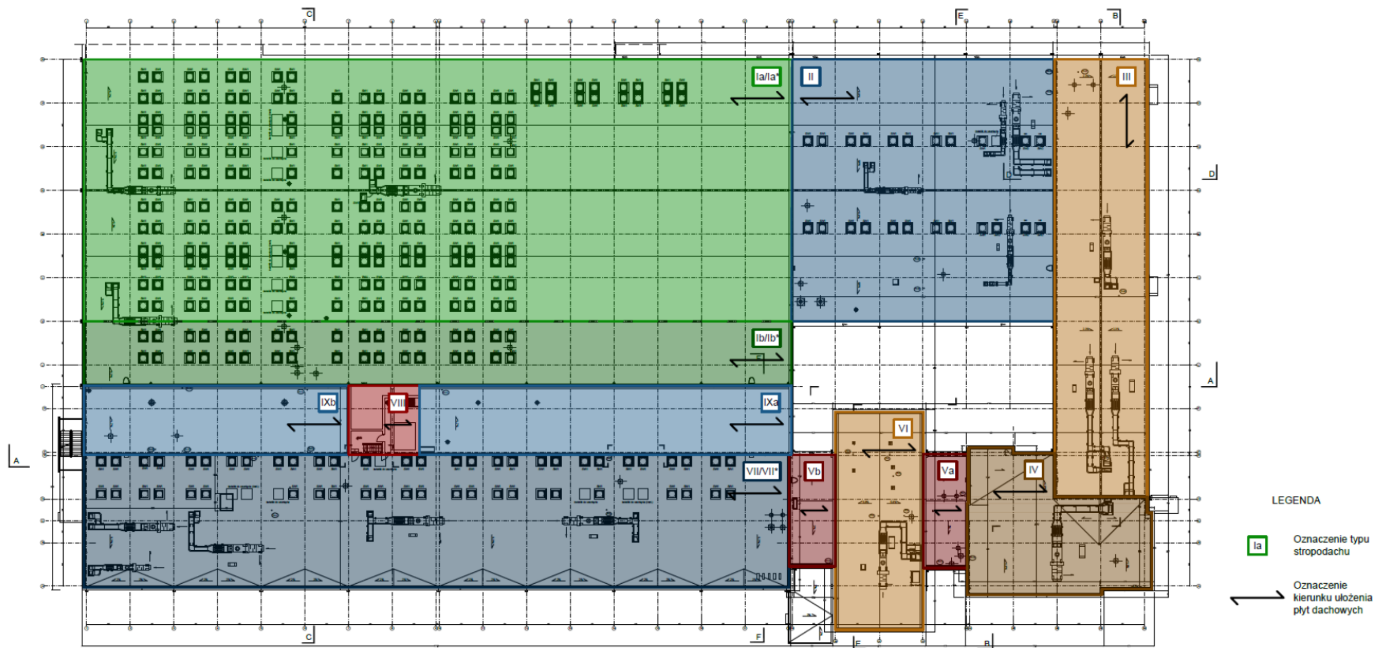
Rzut dachu budynku „C” z oznaczeniem charakterystycznych obszarów
