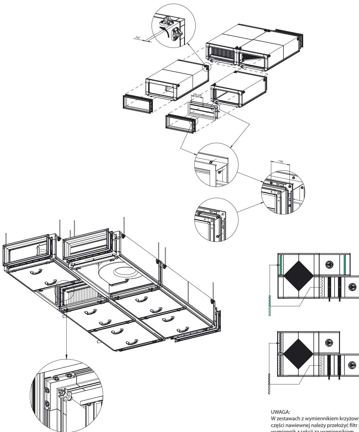
Rys.10 Łączenie sekcji i montaż elementów opcjonalnych
