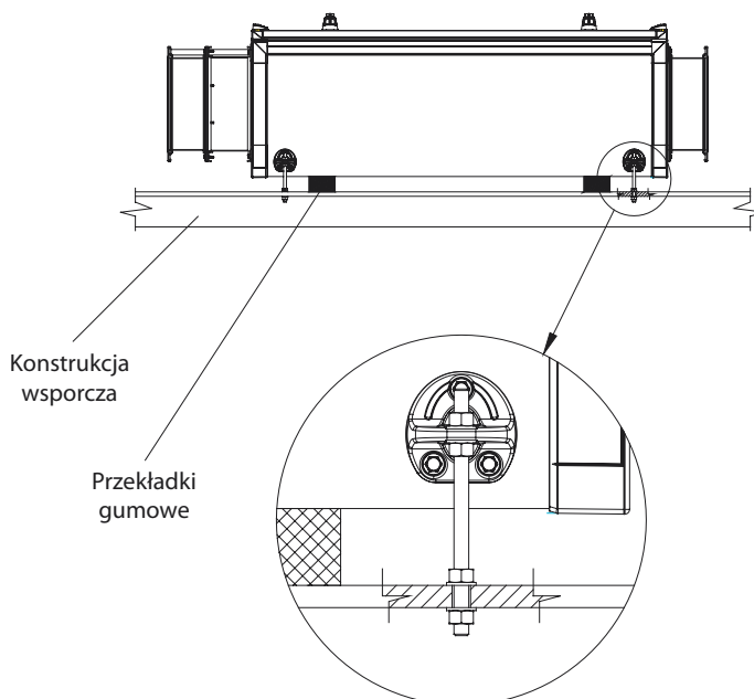
Rys.8 Przykład posadowienia w pozycji leżącej
