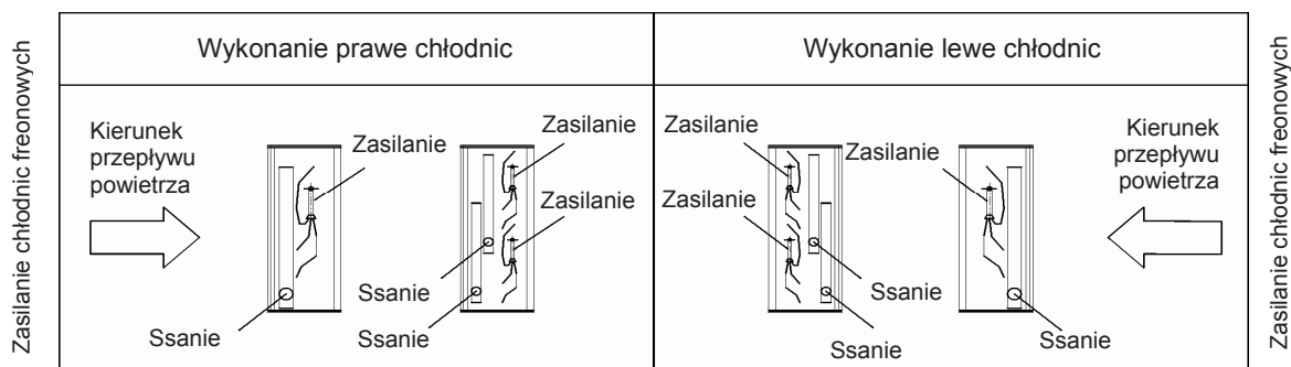
Rys. 18 Zasilanie chłodnic freonowych
