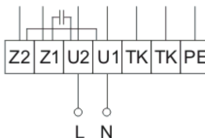
Rys.23 Schemat podłączenia silnika w urządzeniu VS 10 i VS 15
