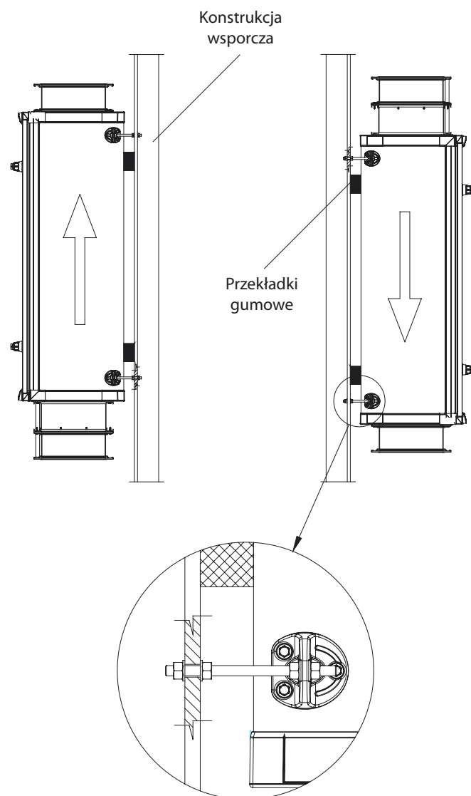
Rys.9 Przykład posadowienia w pozycji pionowej
