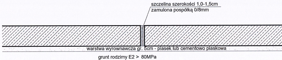
Rys.1 schemat ułożenia płyt drogowych
